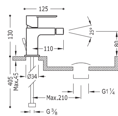
Egykaros bidé csaptelep 200.120.01.D 46 690 Ft
