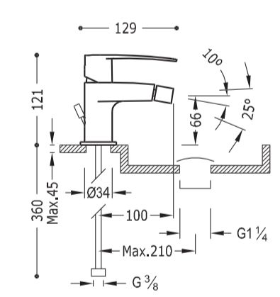
Egykaros bidé csaptelep 204.120.01.D 25 490 Ft
