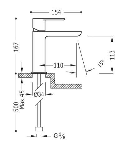
Egykaros mosdó csaptelep, cascade kifolyással 200.101.01 45 990 Ft
