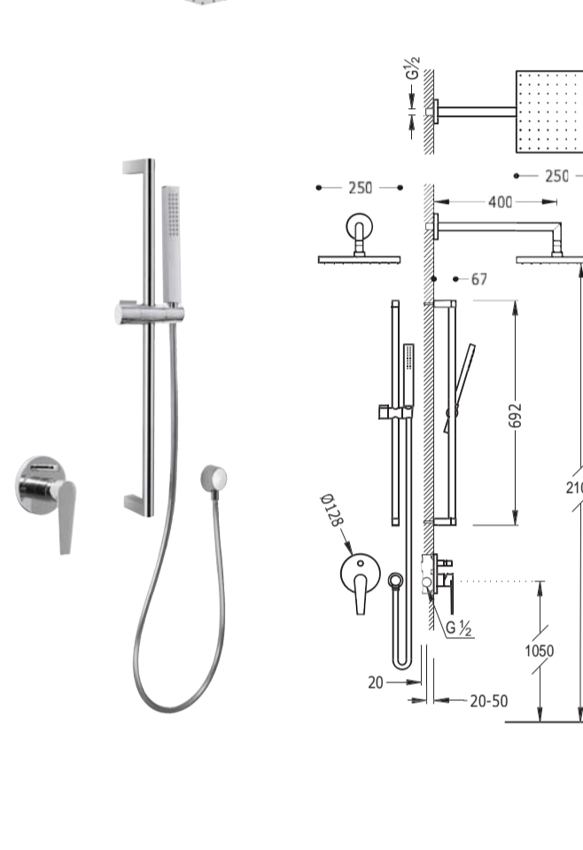
Falba épített zuhanyoztett, zuhanyváltóval + kézi zuhanyoztett + tartó rúd 205.180.05 121 690 Ft
