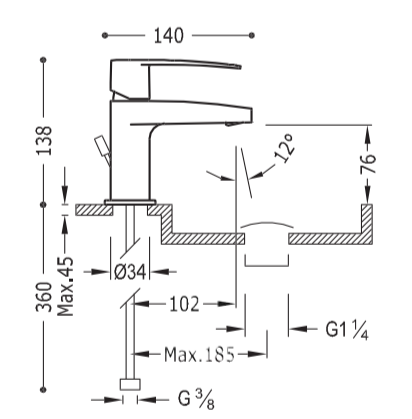
Egykaros mosdó csaptelep leeresztővel 204.103.01.D 25 190 Ft
