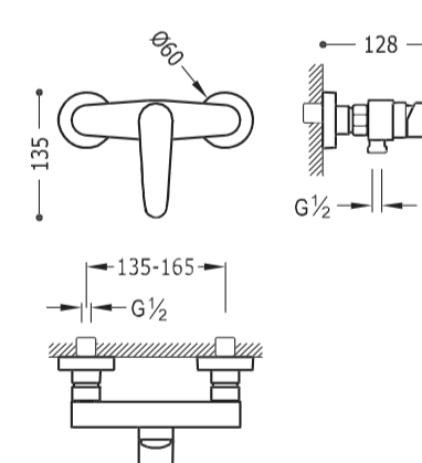
Egykaros zuhany csaptelep + kézi zuhanyoztett 204.167.01 33 890 Ft
