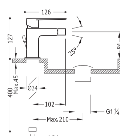
Egykaros bidé csaptelep 205.120.01.D 37 390 Ft
