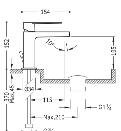
Egykaros mosdó csaptelep leeresztővel 205.103.01.D 37 390 Ft
