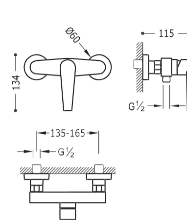
Egykaros zuhany csaptelep 205.167.01 40 090 Ft
